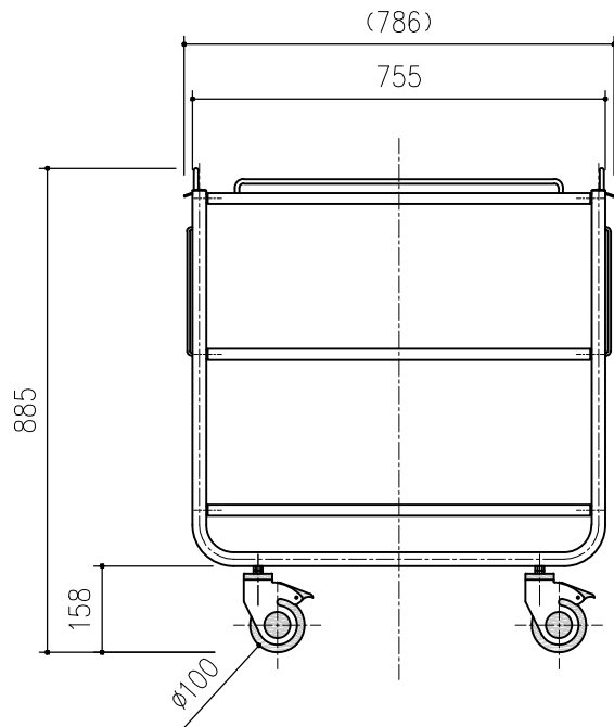
Smart_Wagon_Front_3PT
