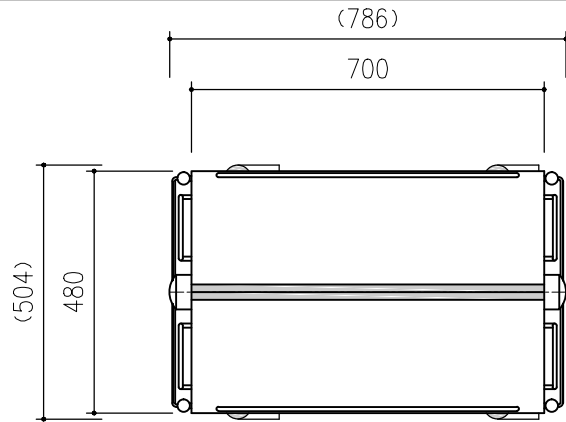
Smart_Wagon_Upper_3PT
