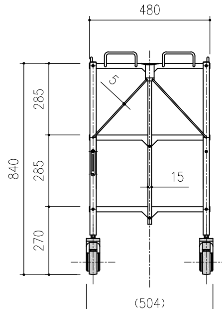
Smart_Wagon_Side_3PT
